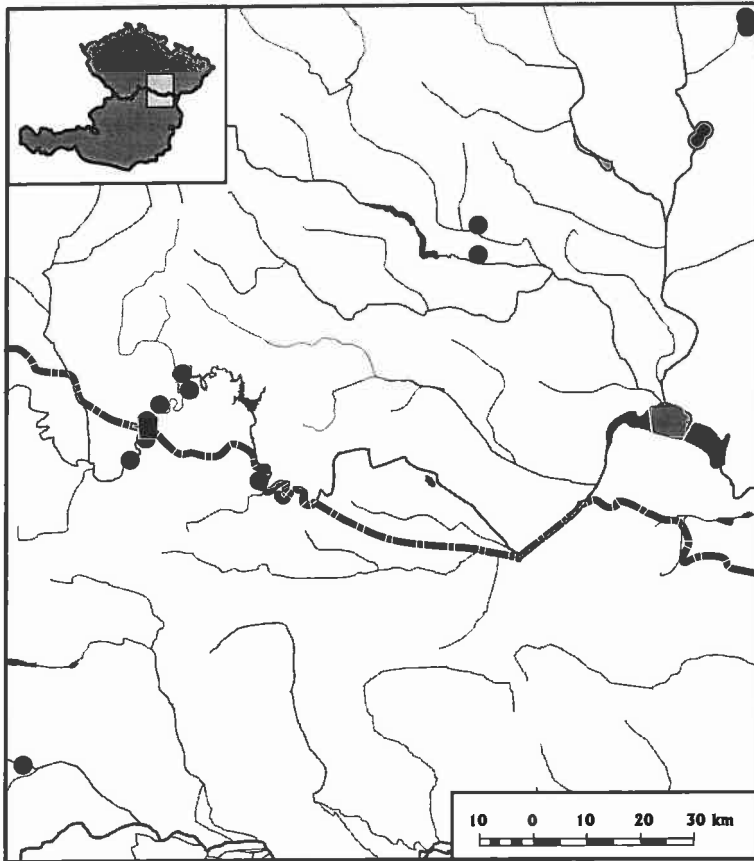
Abb. 2: Verbreitung des Centaureo stoebes-Allietum montani am Südostrand der Böhmischen Masse.
